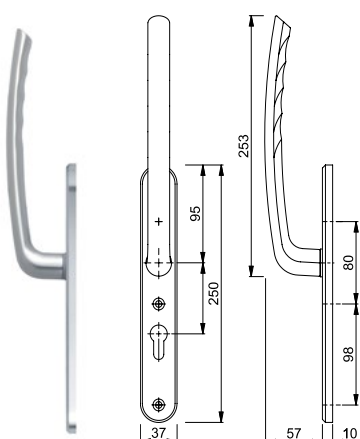
328690 / 328692
